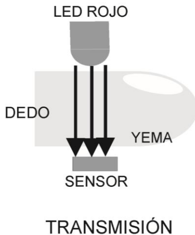
Fig. 1. Adquisición de la señal de pulso oximetría: transmisión y reflexión. Fuente: autores.
