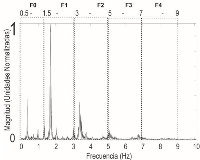
Fig. 5. Magnitud del espectro en potencia de la señal SPO2. Fuente: autores.
