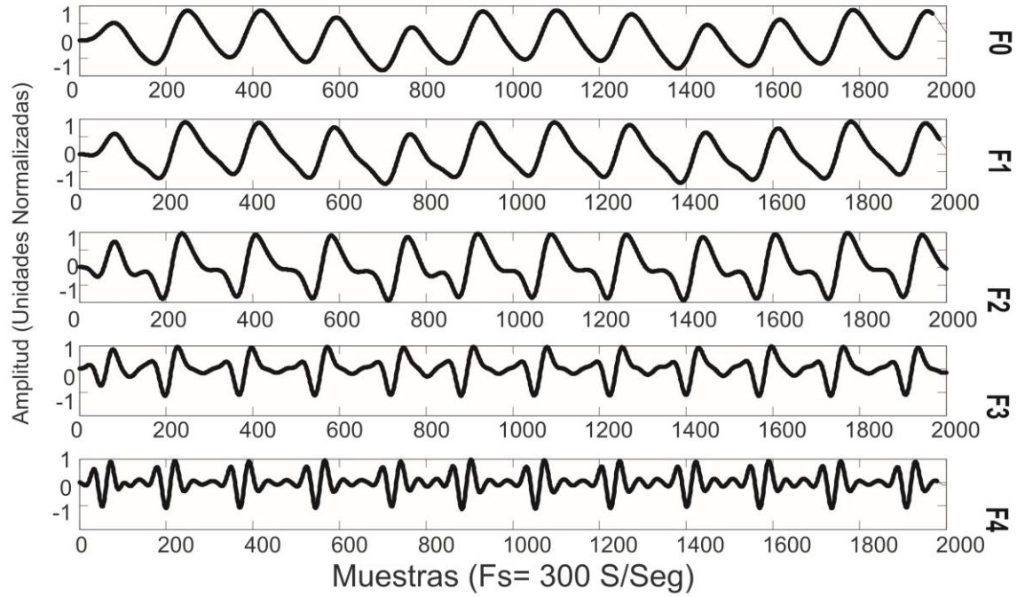
Fig. 9. Resultado de la ejecución del banco de filtros. Fuente: autores.
