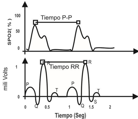
Fig. 2. Señal de pulso oximetría y el electrocardiograma. Fuente: autores.
