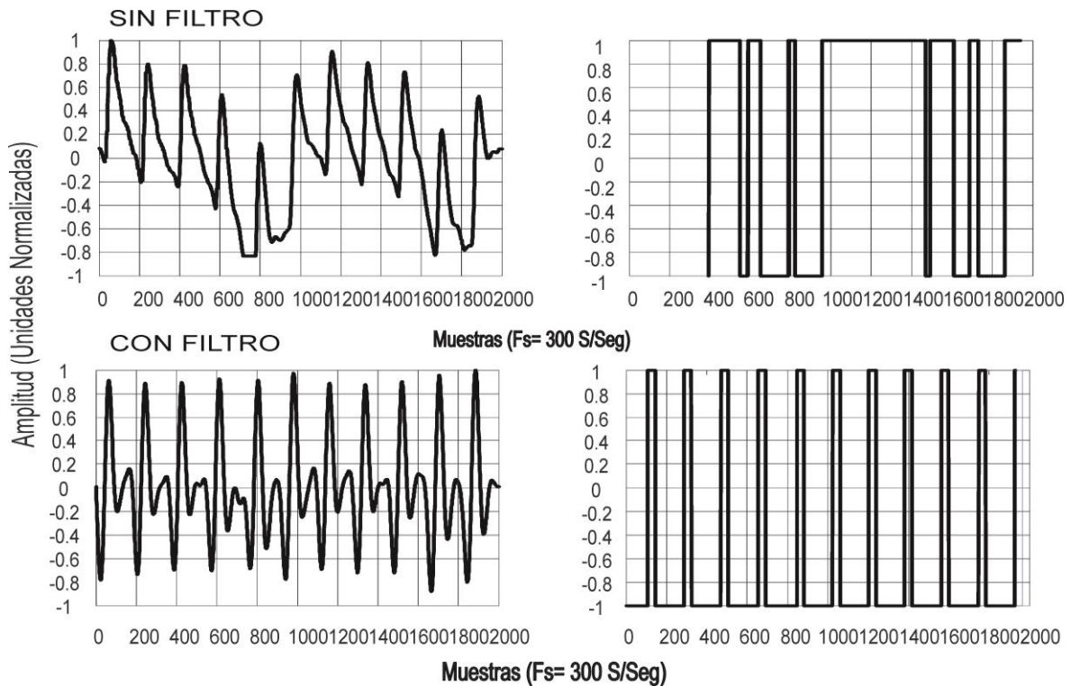
Fig. 13. Comparación del uso del filtro pasa banda en el proceso de umbralización. Fuente: autores.
