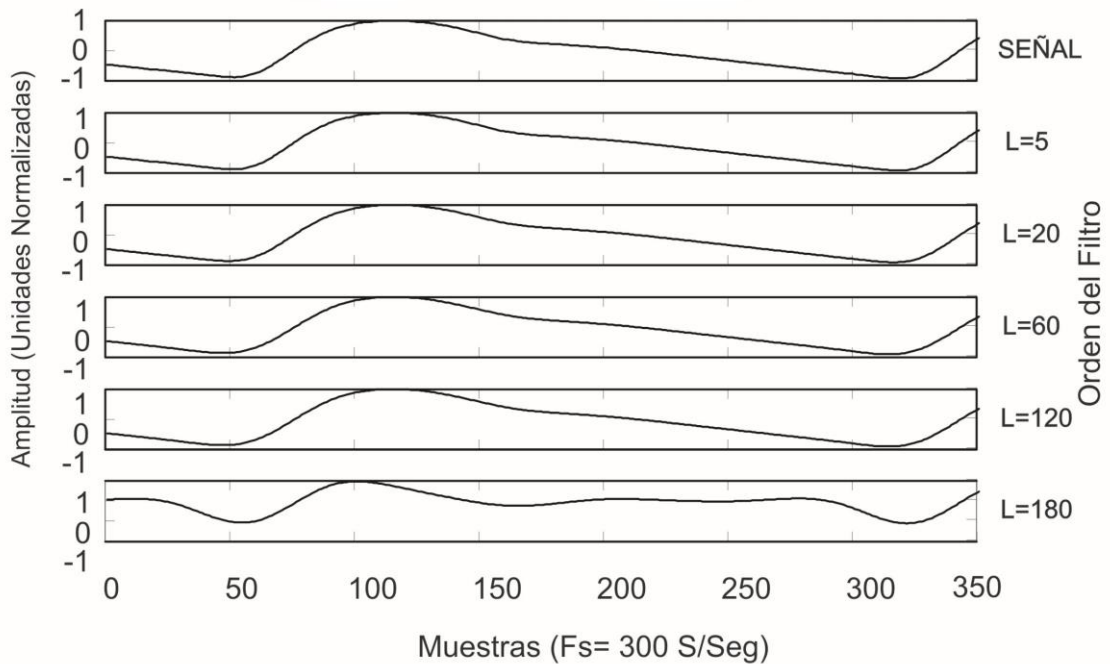
Fig. 10. Prueba de orden del Filtro. Fuente: autores.
