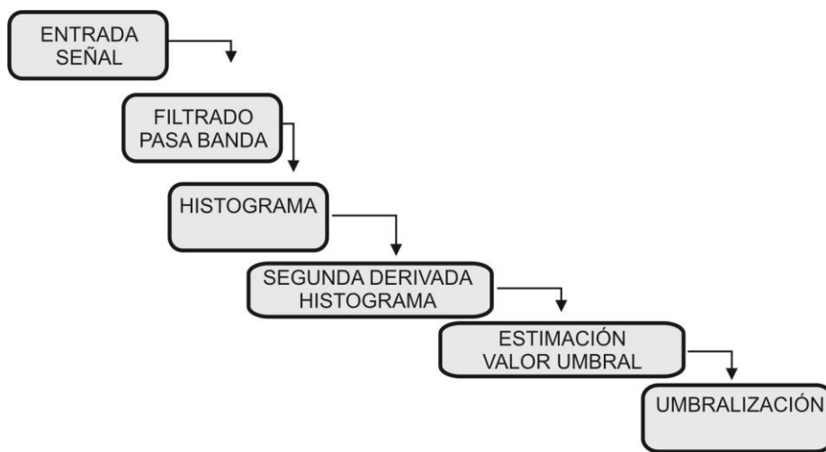
Fig. 8. Umbralización señales ECG y PPG. Fuente: autores.
