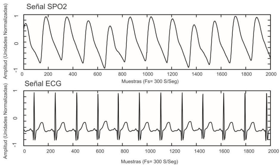
Fig. 4. Señal SPO2 y ECG adquiridas simultáneamente. Fuente: autores.
