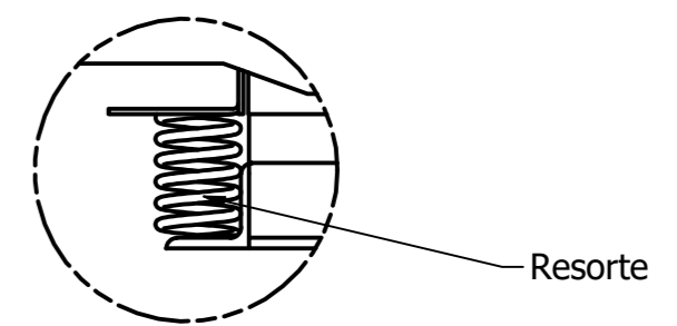
DETALLE Detalle A ESCALA 0,40 : 1
