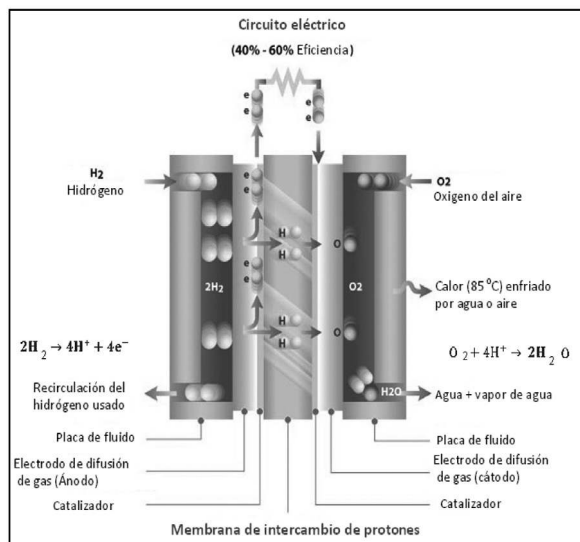
Ilustración 5: Principio de funcionamiento de una celda de combustible adaptada de [Ballard, 2010], [Kruger, 2006]
