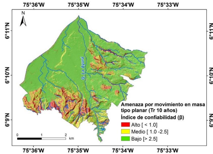
Fig. 8. Índice de confiabilidad– Periodo de retorno 10 años. Fuente: autores.
