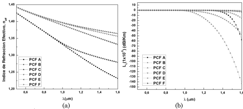
Fig. 2. (a) Índice efectivo n_{eff} y (b) factor de pérdidas por confinamiento L_c para las diferentes configuraciones de PCF's
