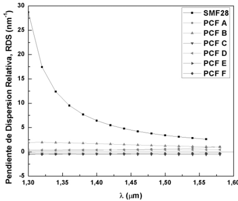
Fig. 4. RDS de la fibra después de la compensación empleando las diferentes PCF propuestas en el trabajo
